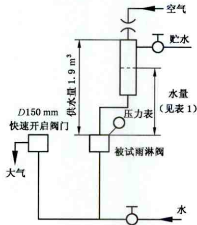
图 3 防复位试验
